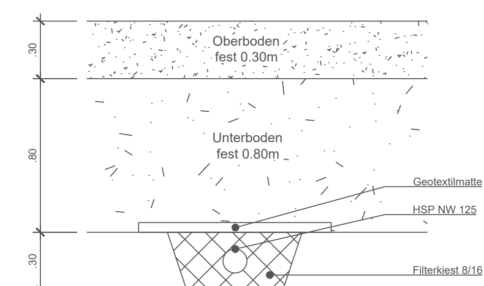
Normalprofil Entwässerung, 1:20
